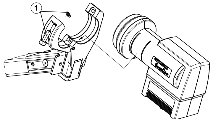
Abb. 5: Speisesystemhalterung montieren
