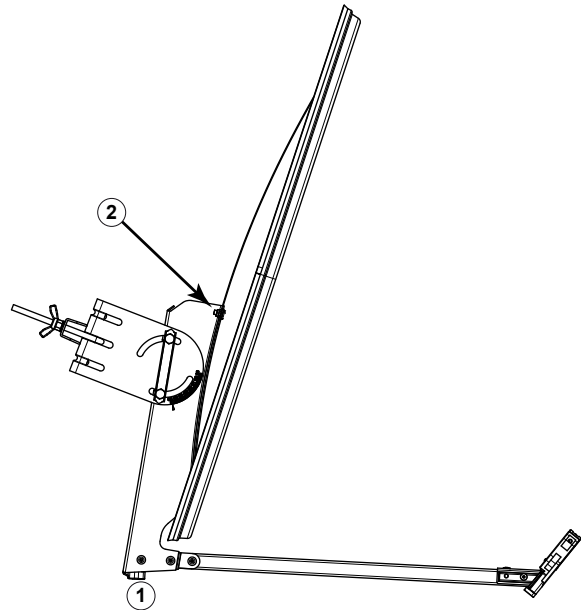
Abb. 4: Reflektor montieren
