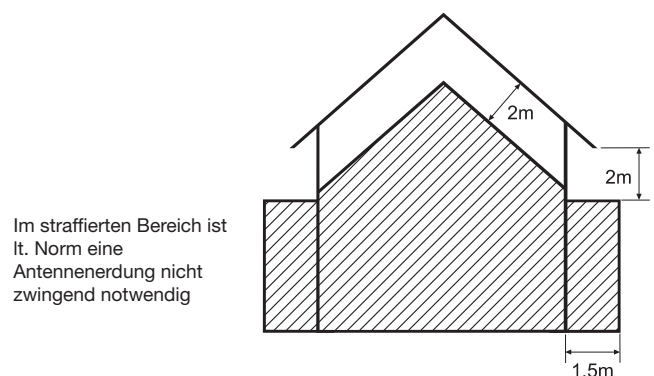
Abb. 13: Bereiche für Antennen- und Blitzschutzanlage
