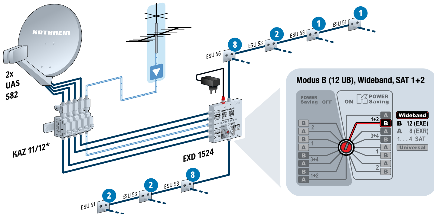
UAS 582 mit Einkabel-Multischalter EXD 1524
