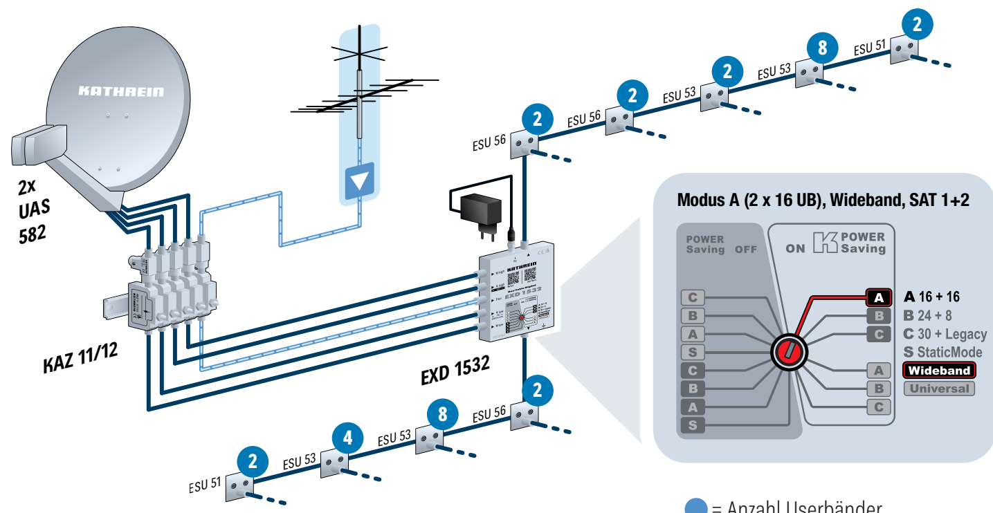
UAS 582 mit Einkabel-Multischalter EXD 1532
