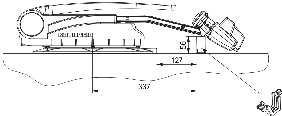
Tragarm-Stütze montieren
