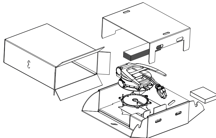
Dreheinheit auspacken
