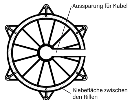
Kleber aufbringen
