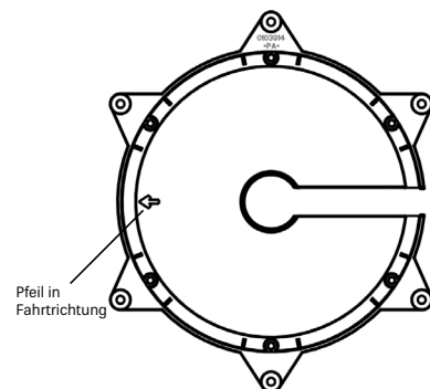
Montageplatte ausrichten
