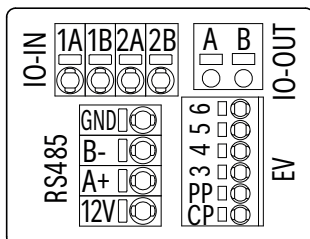
Benutzerschnittstellen
