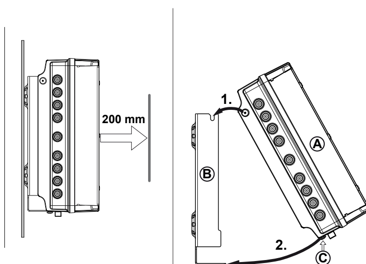
Abb. 3: Kopfstelle einhängen
