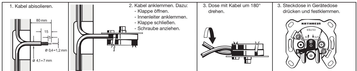
Abb. 3: Steckdosen montieren
